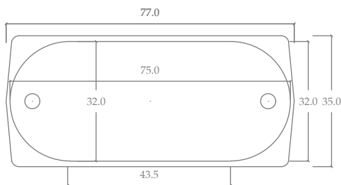
Boitier d'encastrement
